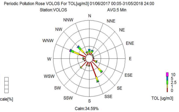
Τολουόλιο ( \mu\text{g}/\text{m}^3 )
