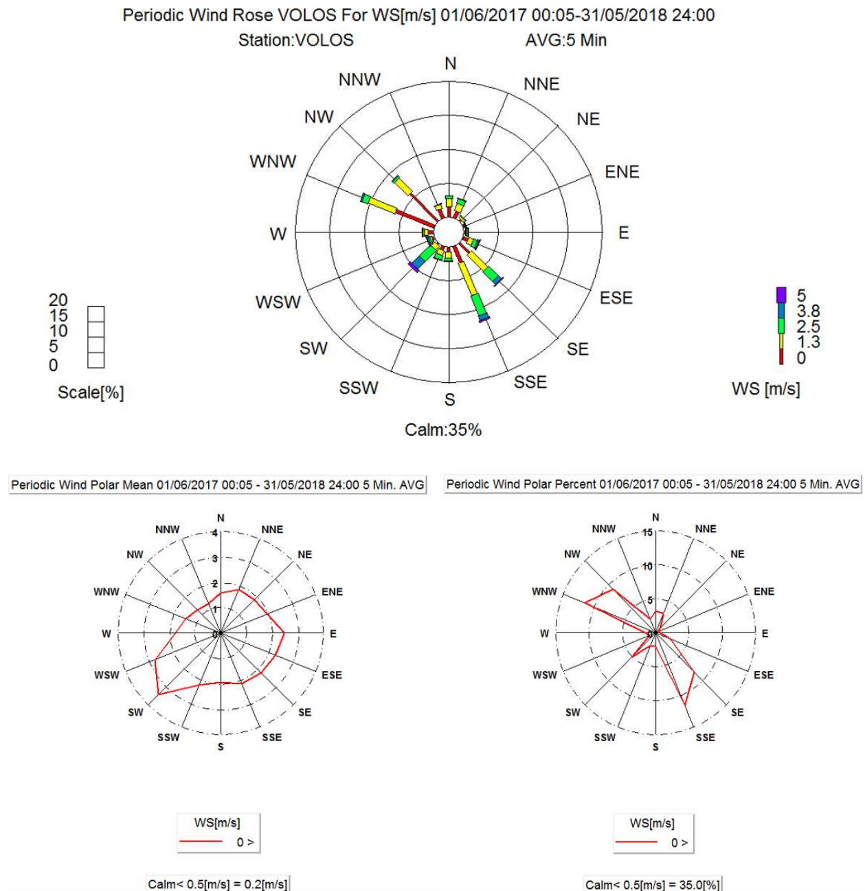
Σχήμα 2.1.4. Επάνω: Ροδογράμματα επικρατούντων ανέμων κατά την περίοδο των μετρήσεων Κάτω: Μέση ταχύτητα ανέμου ανά διεύθυνση προέλευσης
