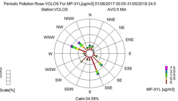
m,p- Ξυλόλιο ( \mu\text{g}/\text{m}^3 )
