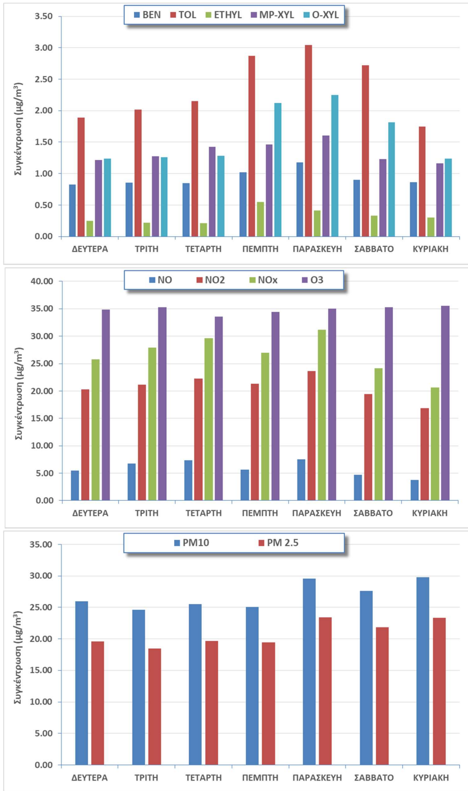
Σχήμα 2.1.2. Μέση εβδομαδιαία διακύμανση των συγκεντρώσεων BTEX, NO x , O 3 , PM 10 και PM 2.5 κατά το χρονικό διάστημα 02/06/2017 – 01/06/2018
