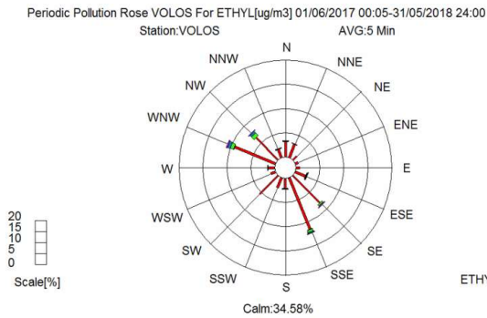
Αιθυλο-Βενζόλιο ( \mu\text{g}/\text{m}^3 )
