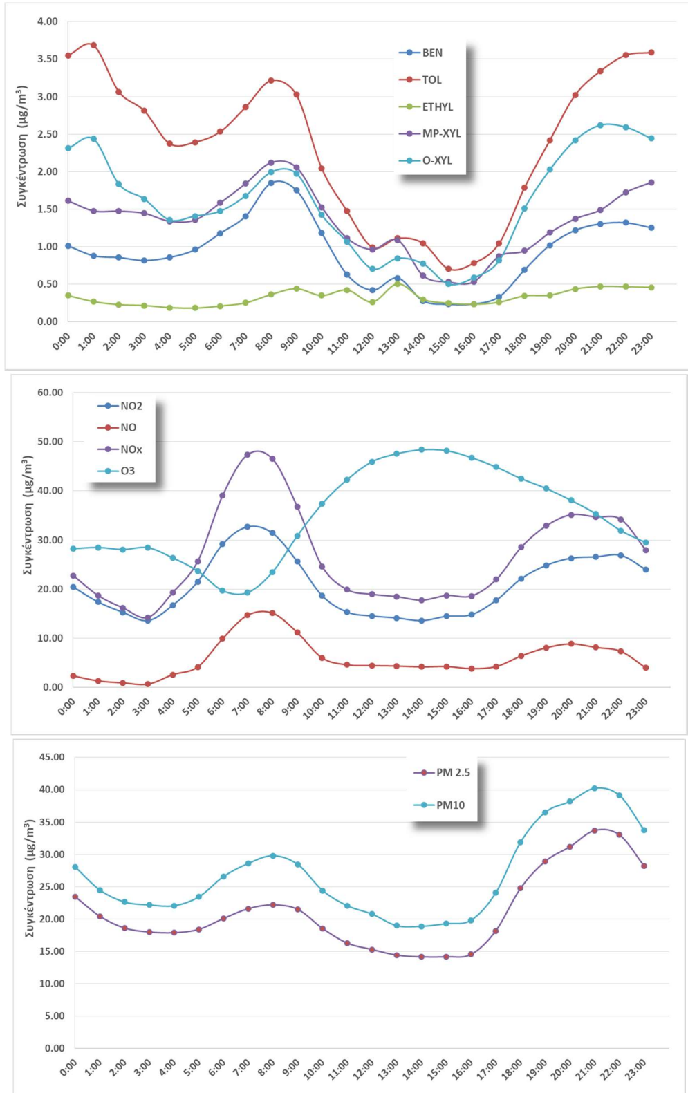
Σχήμα 2.1.1. Μέση ημερήσια διακύμανση των συγκεντρώσεων BTEX, NO x , O 3 , PM 10 και PM 2.5 κατά το χρονικό διάστημα 02/06/2017 – 01/06/2018
