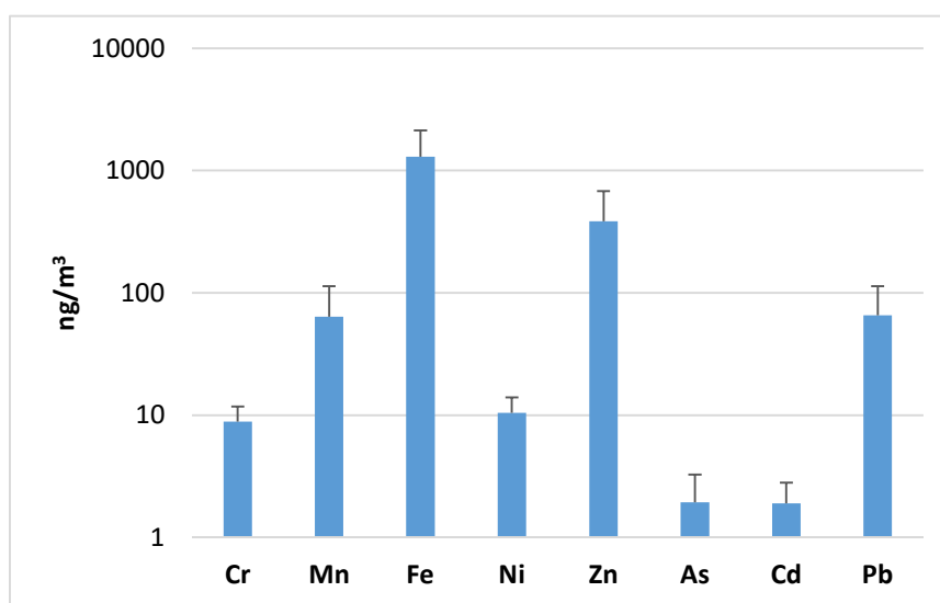
Σχήμα 2.2.3. Μέση τιμή και τυπική απόκλιση της συγκέντρωσης μετάλλων/μεταλλοειδών κατά το χρονικό διάστημα 02/06/2017 – 01/06/2018
