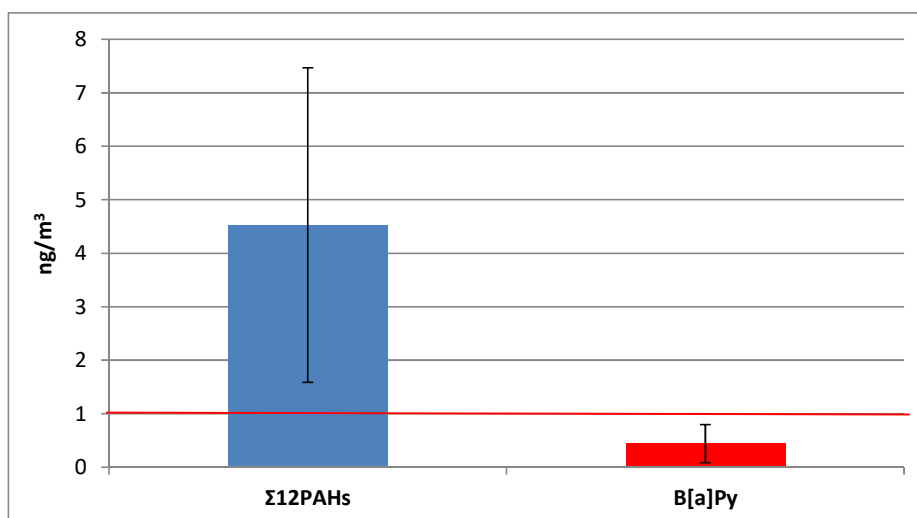
Σχήμα 2.2.3. Μέση τιμή και τυπική απόκλιση της συνολικής συγκέντρωσης Σ12PAHs και του B[a]Py κατά το χρονικό διάστημα 02/06/2016 – 01/06/2017
