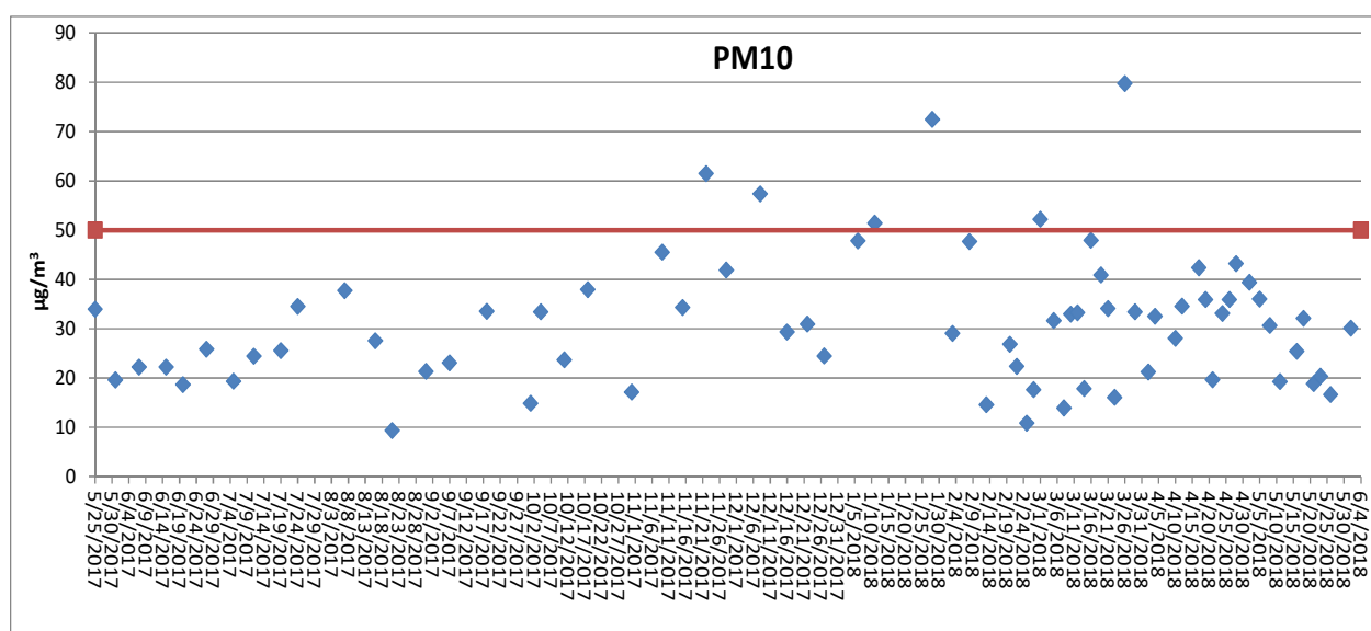
Σχήμα 2.2.1. Ημερήσιες σταθμικές συγκεντρώσεις PM10 κατά το χρονικό διάστημα 02/06/2017 – 01/06/2018
