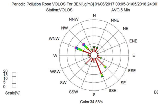
Βενζόλιο ( \mu\text{g}/\text{m}^3 )
