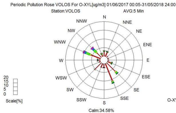
ο- Ξυλόλιο ( \mu\text{g}/\text{m}^3 )
