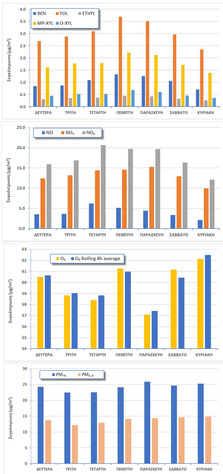
Σχήμα 2.1.2. Μέση εβδομαδιαία διακύμανση των συγκεντρώσεων BTEX, NO x , O 3 , κυλιόμενου δωρου μ.ο. O 3 , PM 10 και PM 2.5 κατά το χρονικό διάστημα 01.06.22 – 30.11.22
