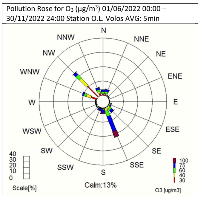
Σχήμα 2.1.5. Ροδογράμματα των συγκεντρώσεων των αρωματικών υδρογονανθράκων BTEX, NO, NO 2 , NO x , O 3 και PM 10 (5-15 min Average)
