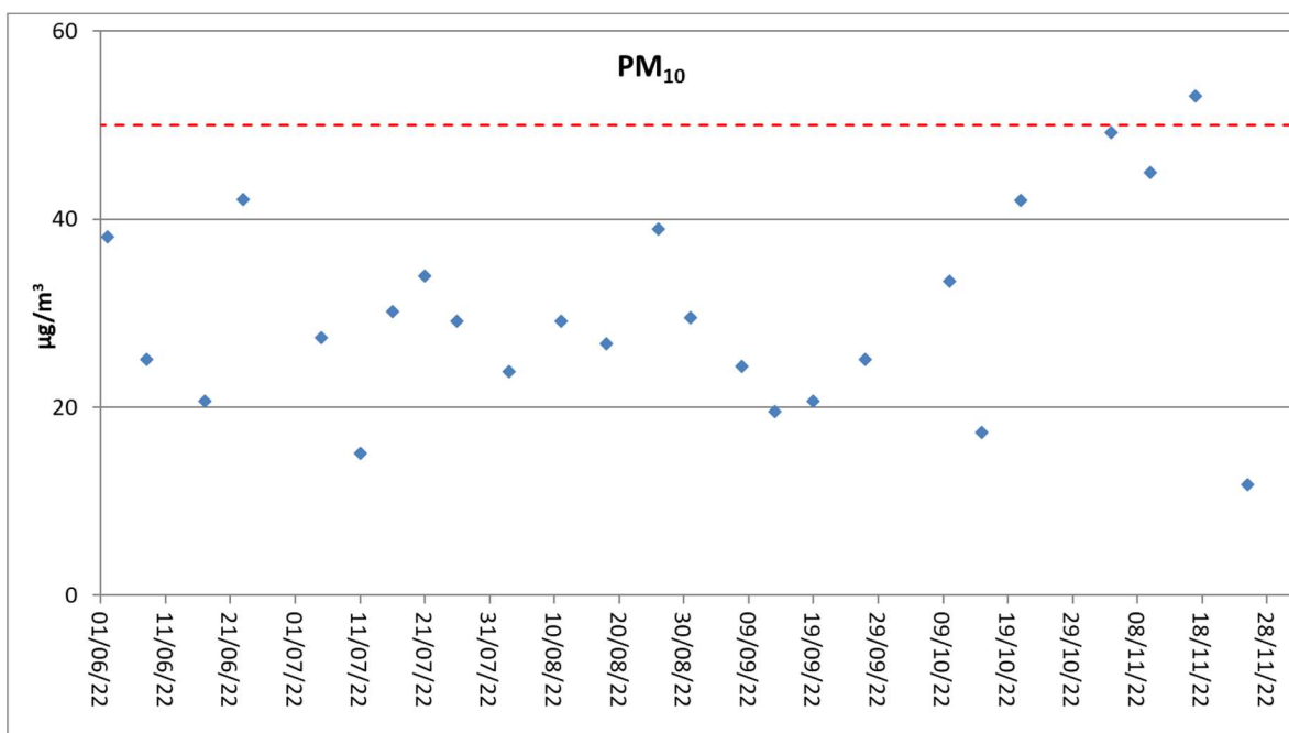
Σχήμα 2.2.1. Ημερήσιες σταθμικές συγκεντρώσεις PM 10 κατά το χρονικό διάστημα 01.06.22 – 30.11.22
