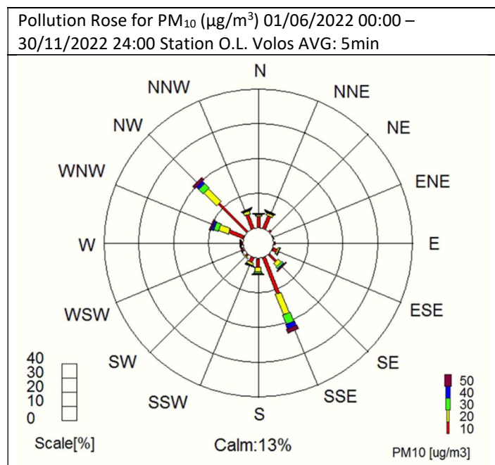
Σχήμα 2.1.5. Ροδογράμματα των συγκεντρώσεων των αρωματικών υδρογονανθράκων BTEX, NO, NO 2 , NO x , O 3 και PM 10 (5-15 min Average)
