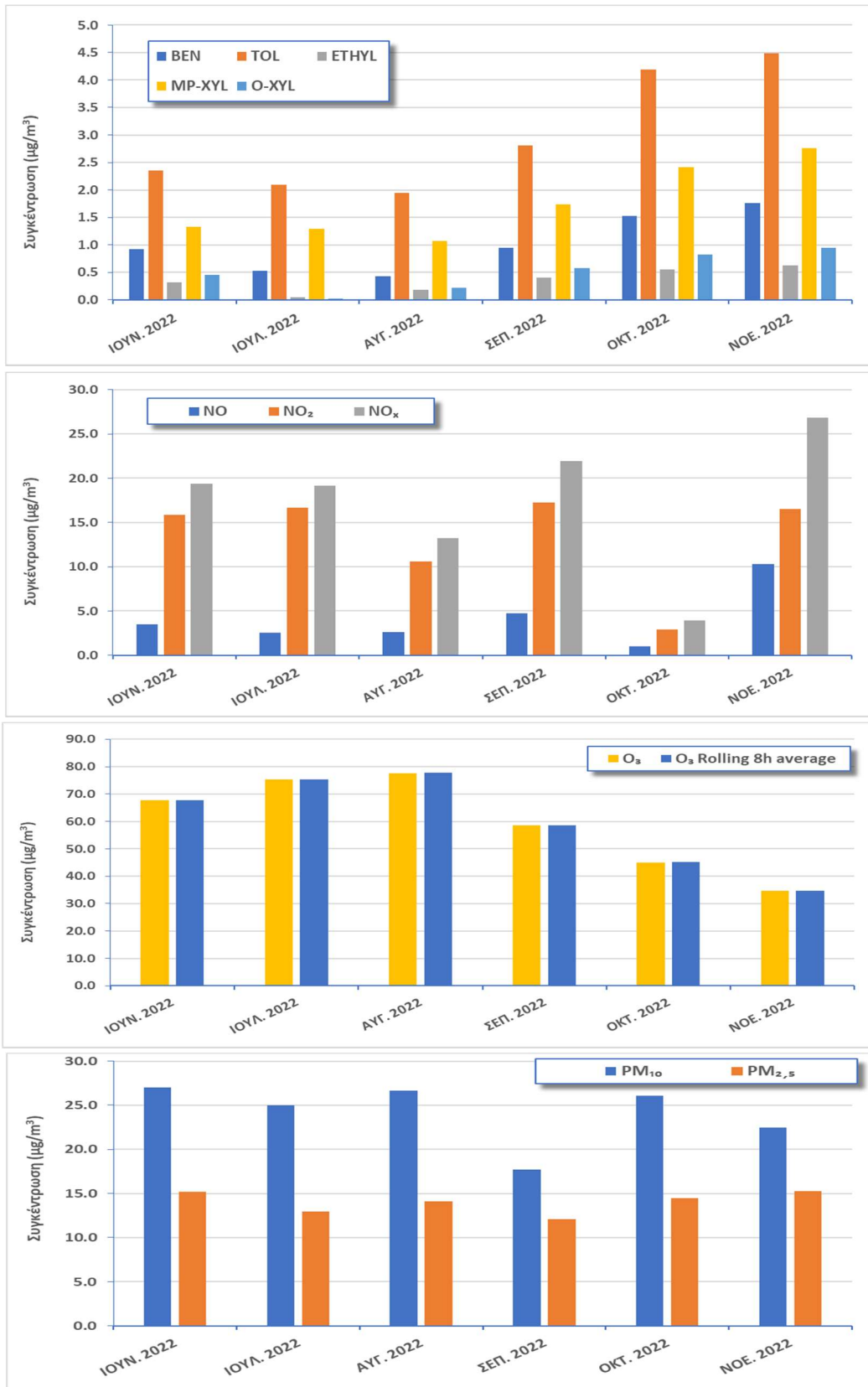
Σχήμα 2.1.3. Μέση μηνιαία διακύμανση των συγκεντρώσεων BTEX, NO x , O 3 , κυλιόμενου δρωρου μ.ο. O 3 , PM 10 και PM 2,5 κατά το χρονικό διάστημα 01.06.22 – 30.11.22
