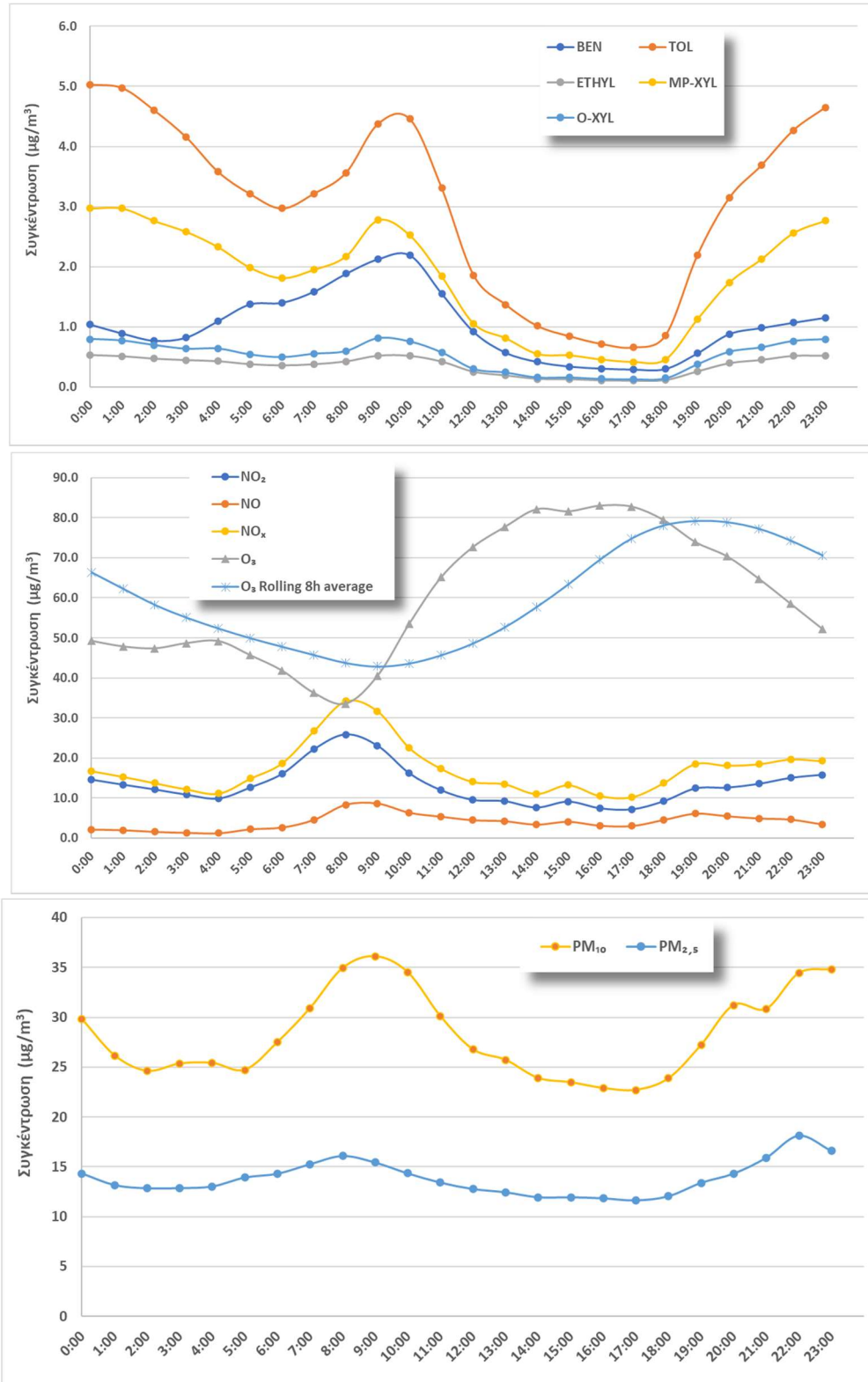
Σχήμα 2.1.1. Μέση ημερήσια διακύμανση των συγκεντρώσεων BTEX, NO x , O 3 , κυλιόμενου δρωρου μ.ο. O 3 , PM 10 και PM 2.5 κατά το χρονικό διάστημα 01.06.22 – 30.11.22
