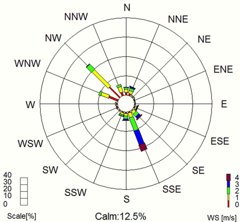
Σχήμα 2.1.4. Συχνότητα εμφάνισης και μέση ταχύτητα ανέμου ανά διεύθυνση προέλευσης κατά την περίοδο των μετρήσεων
