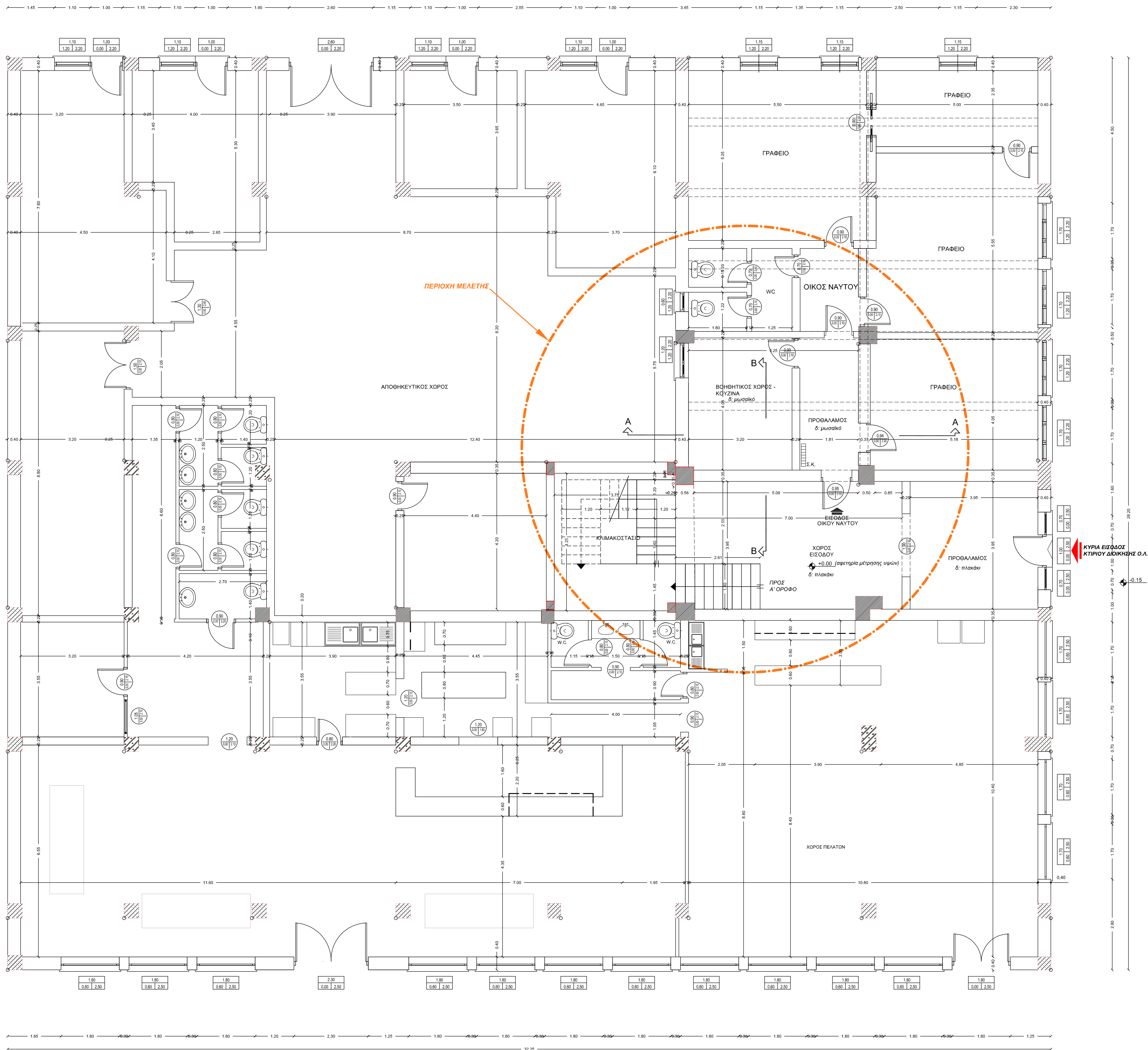
ΚΑΤΟΨΗ ΙΣΟΓΕΙΟΥ
